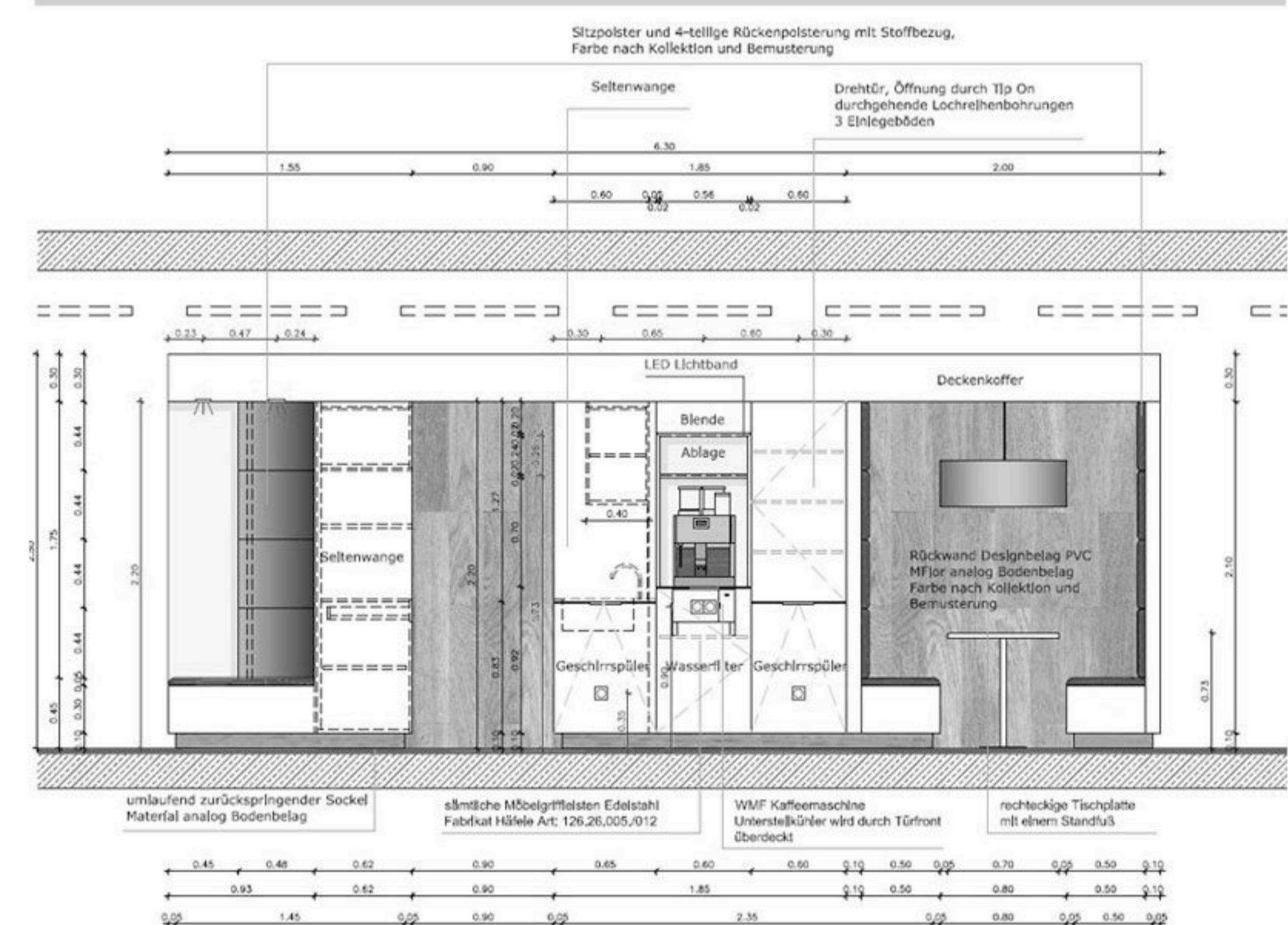
ANSICHT A
